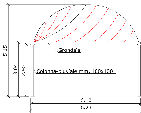
- PROSPETTO
