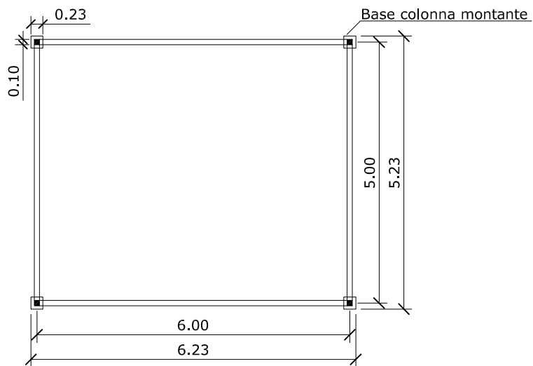
- PIANTA
